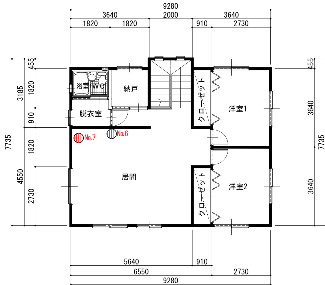
2F平面図 1 : 100
