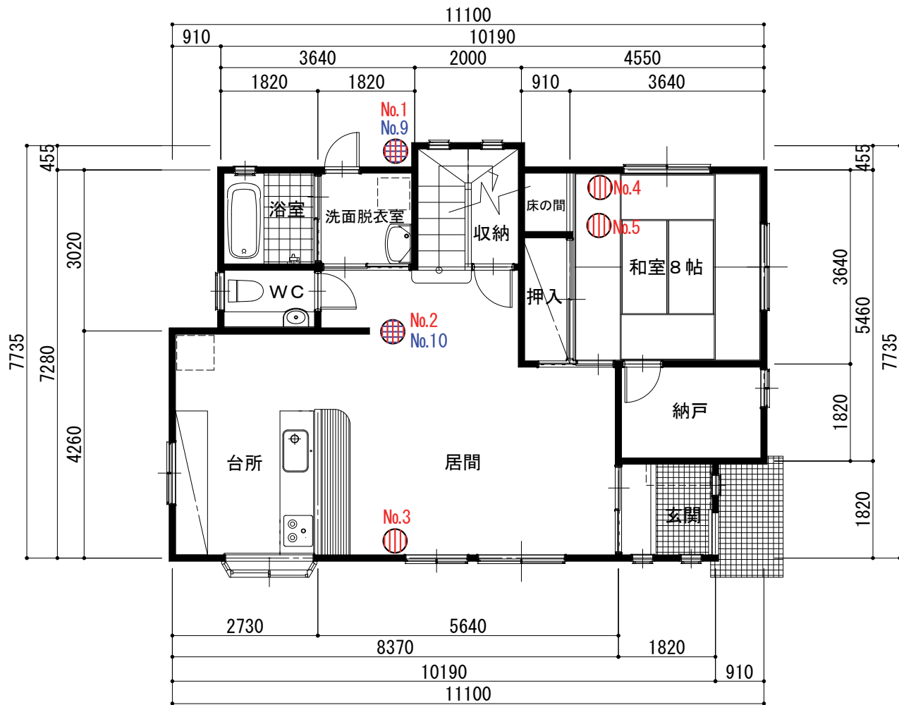
1F平面図 1 : 100
